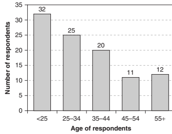
a: one variable (2D)
